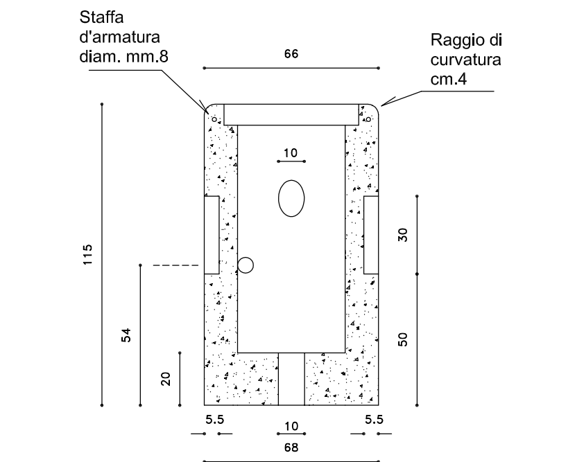
SEZIONE TRASVERSALE
