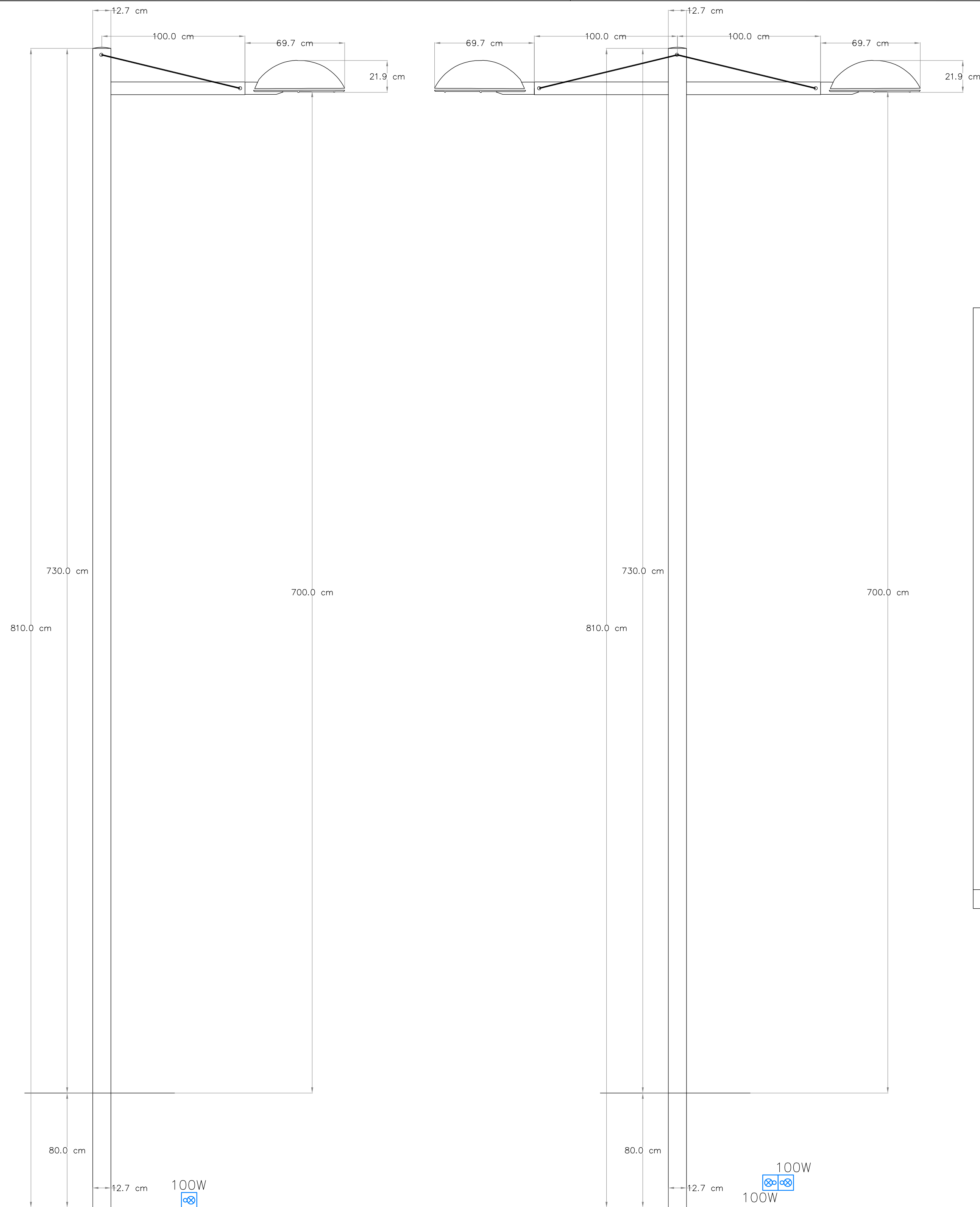
PARTICOLARE CONFORMAZIONE GRUPPO ILLUMINANTE - SCALA 1:20
