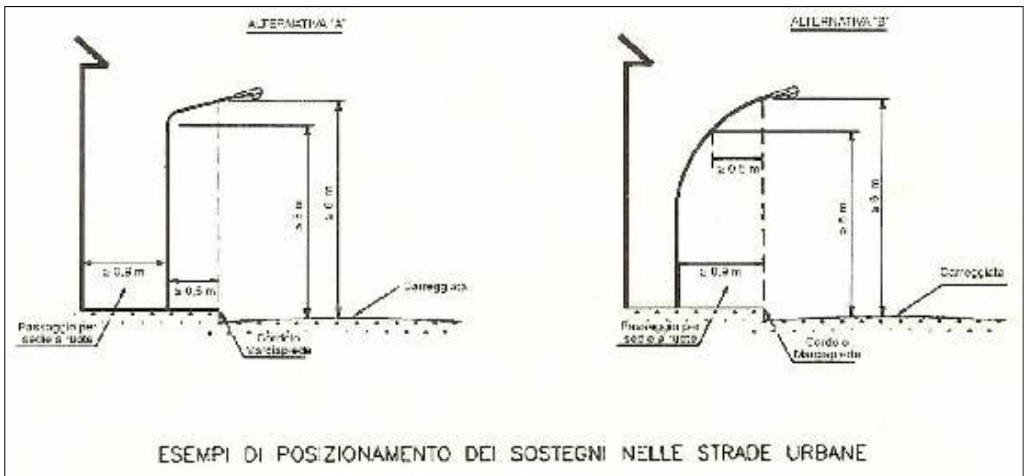
PARTICOLARE DEL DISTANZIAMENTO DEGLI IMPIANTI DAI LIMITI DELLA CARREGGIATA E DALLA SEDE STRADALE
