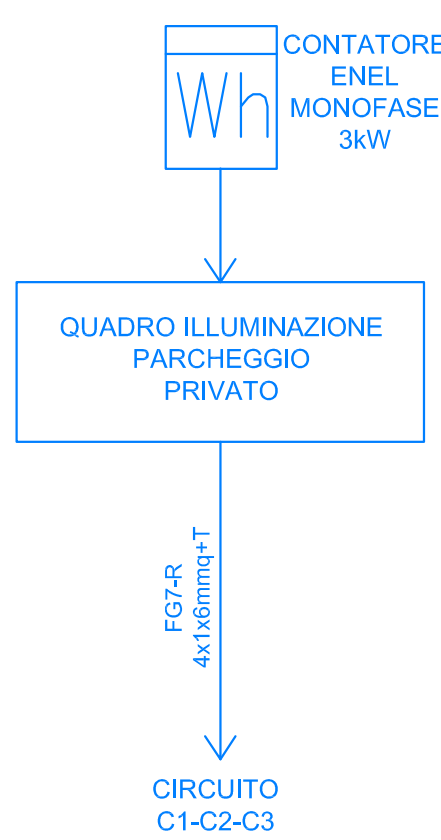
SCHEMI A BLOCCHI IMPIANTO ELETTRICO ILLUMINAZIONE PARCHEGGIO PRIVATO
