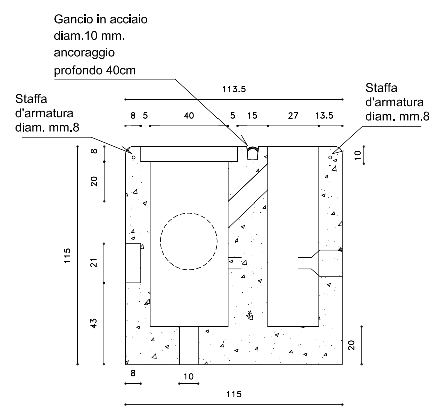
SEZIONE LONGITUDINALE
