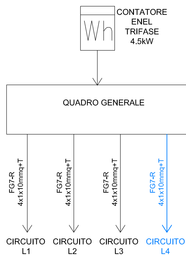
SCHEMI A BLOCCHI IMPIANTO ELETTRICO ILLUMINAZIONE PUBBLICA
