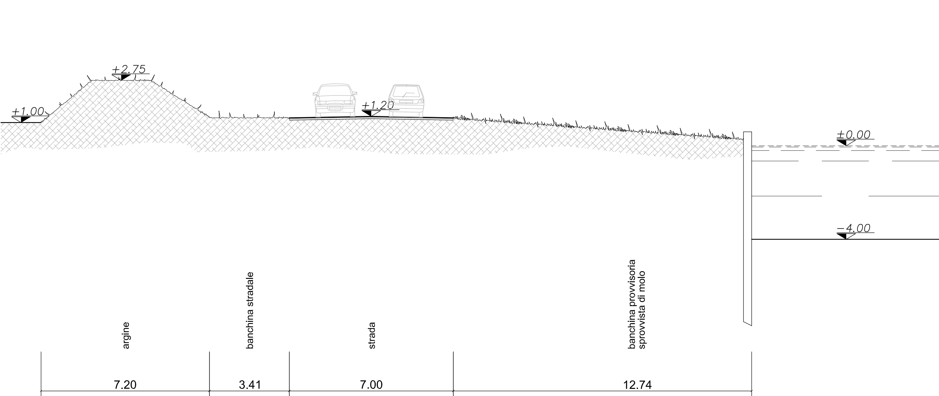
SEZIONE D-D
