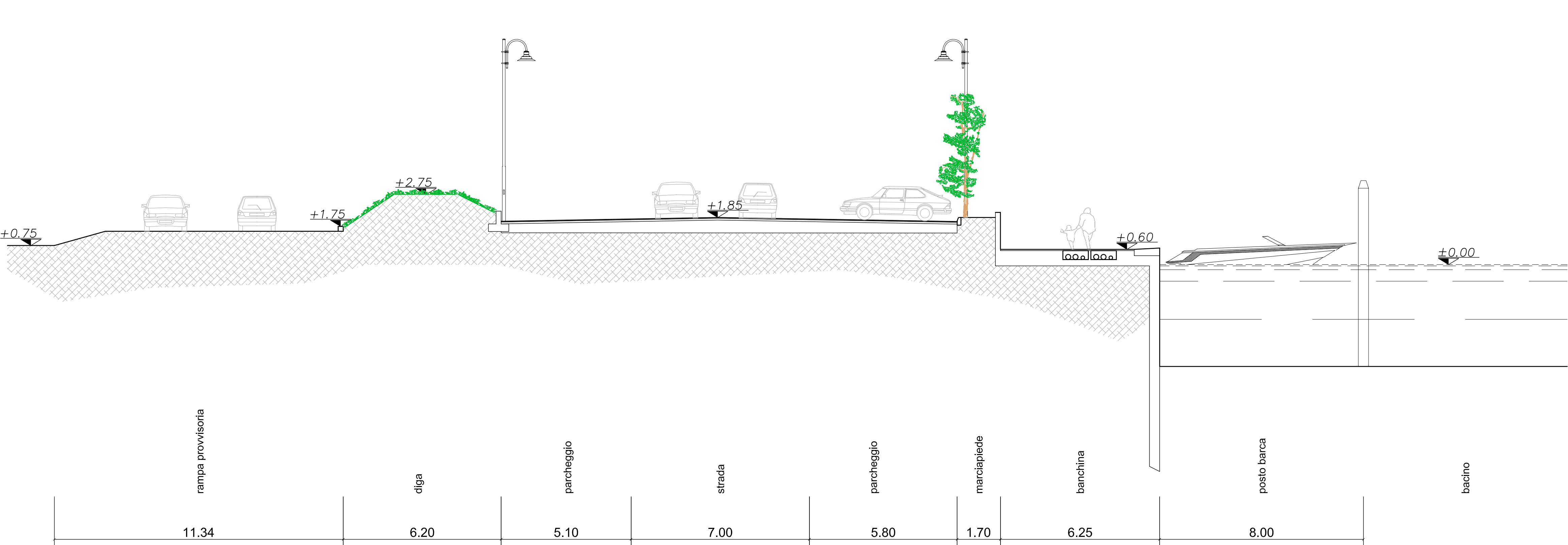
SEZIONE F-F
