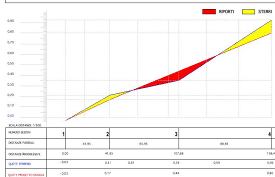
SEZIONI STERRO E RIPORTO
