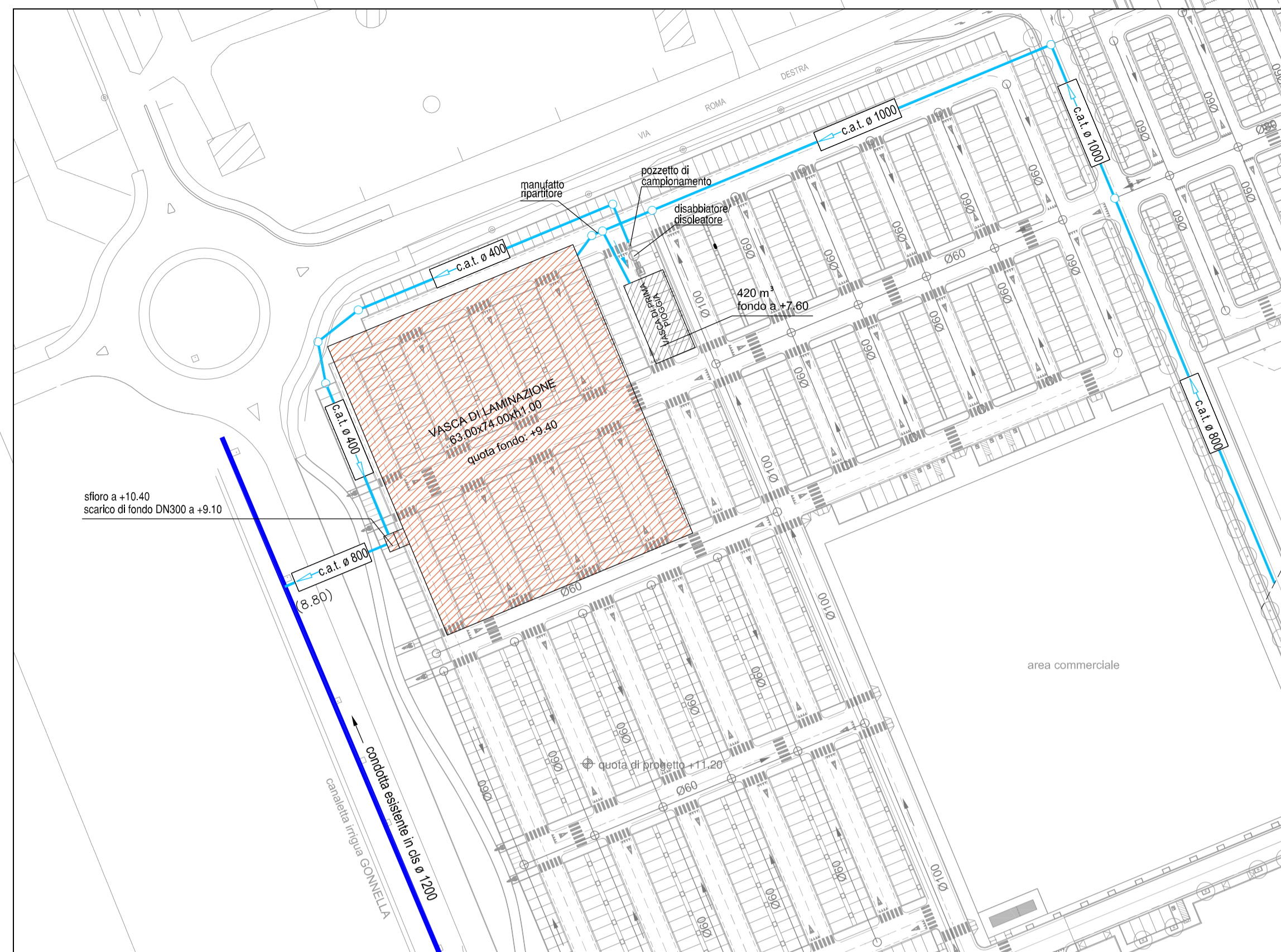
STRALCIO PLANIMETRICO OPERE FOGNARIE RELATIVE ALL'INVARIANZA IDRAULICA - scala 1:1000 (DA REALIZZARSI CONTESTUALMENTE CON IL PUA DELLE DITTE ALI - MARCHETTI E IL PUA DELLE DITTE L' ANCORA - IL SALVAGENTE VERDE - ANCORA COSTRUZIONI COME DA PARERE PROT N. 8049/0,2 IN DATA 13/09/2013 DEL CONSORZIO DI BONIFICA VENETO ORIENTALE)
