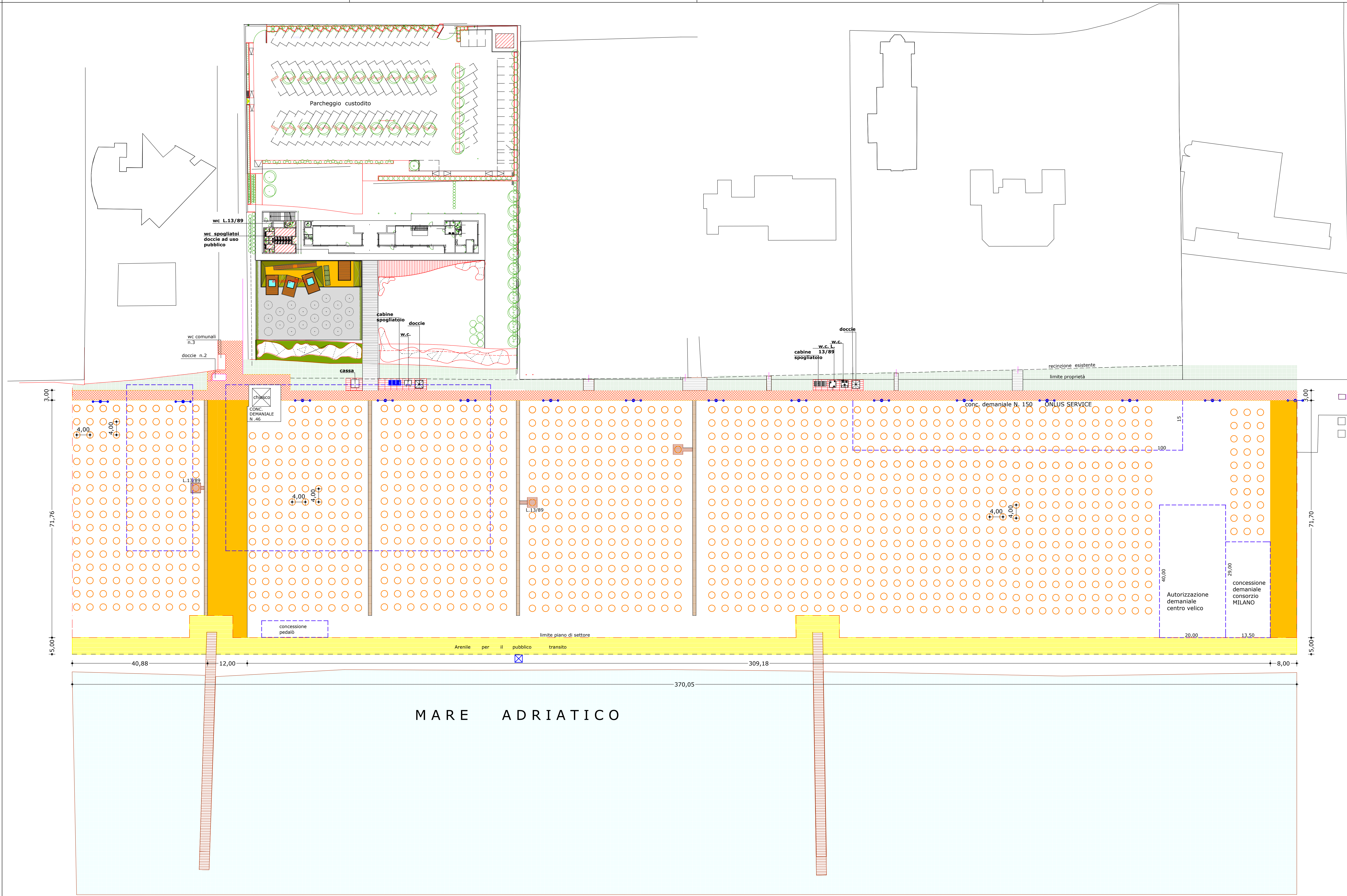
Planimetria generale - STATO AUTORIZZATO Scala 1/500
