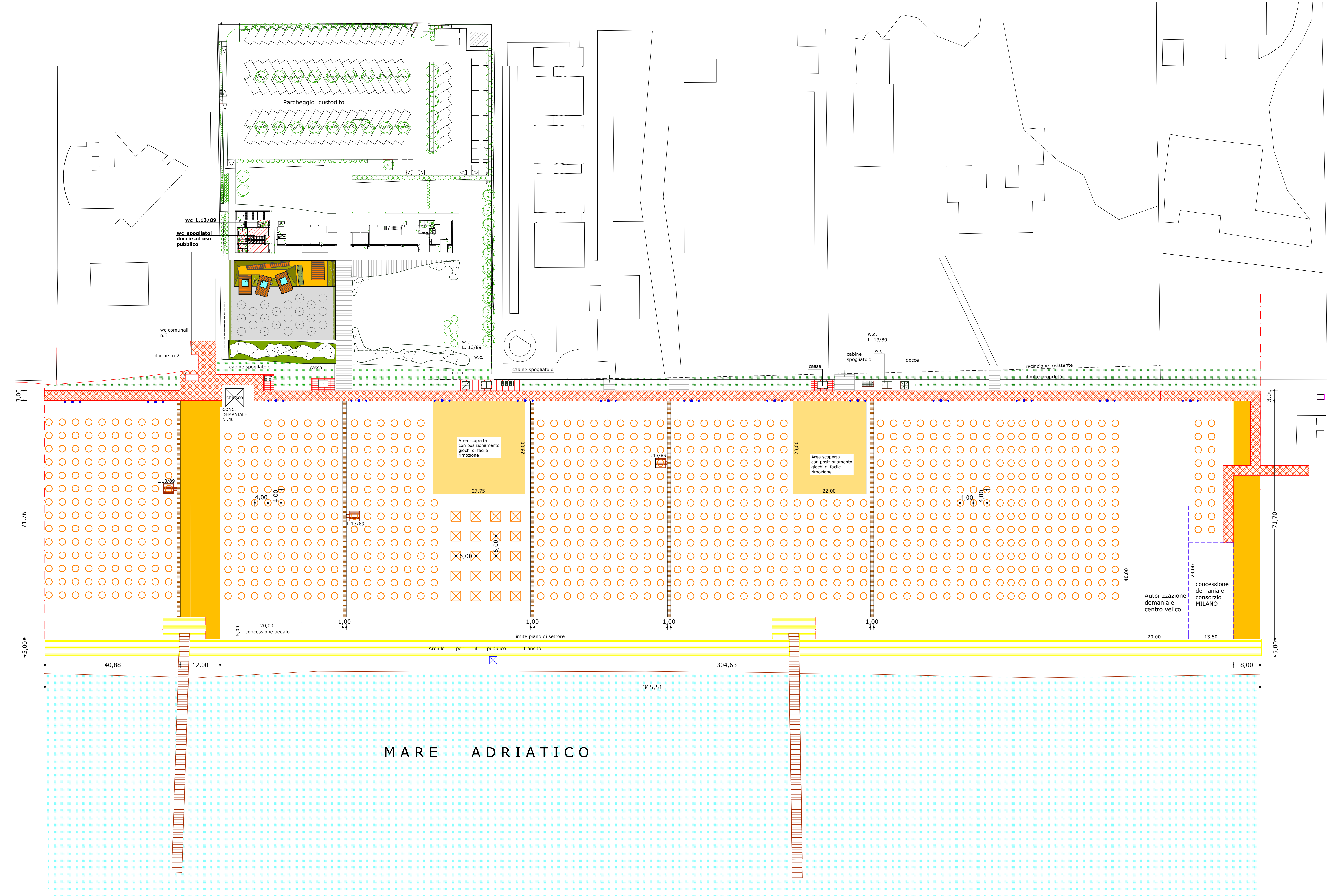
Planimetria generale - STATO DI PROGETTO Scala 1/500
